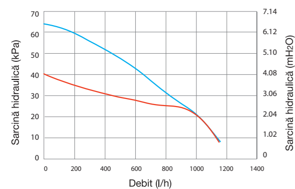
VICTRIX 26 / X 24 Grafic debit / sarcină hidraulică
